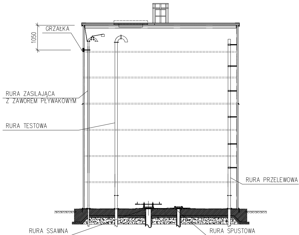
WARIANT PRZYŁĄCZY WYPROWADZONYCH PRZEZ PŁYTĘ FUNDAMENTWA
