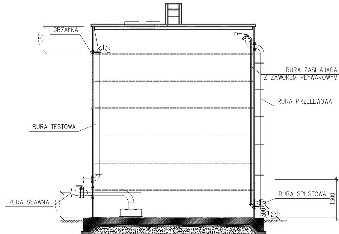
WARIANT PRZYŁĄCZY WYPROWADZONYCH PRZEZ PŁASZCZ ZBIORNIKA
